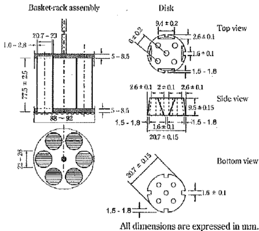
Fig. 6.09-1 Disintegration apparatus
